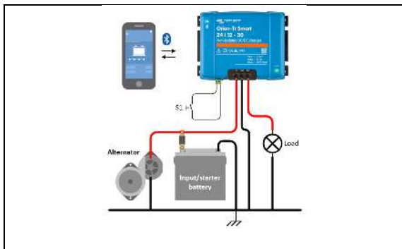
Afbeelding 1: Typische aansluitingsinstelling als DC-DC-omvormer
